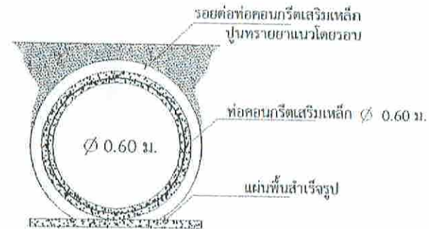
รูปตัดขยาย A
