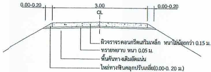
รูปตัดถนนผิวจราจรคอนกรีตเสริมเหล็ก
