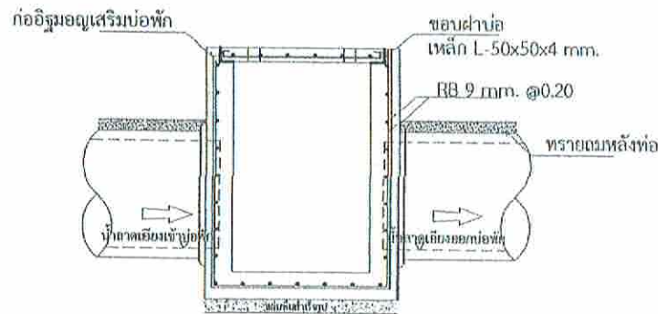
รูปตัดขยายบ่อพักน้ำ B
